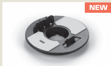
Tête universale fixe Ø 110 mm pour lambourdes en aluminium et en bois Selbstnivellierender UNIVERSAL-Kopf Ø 110 mm für Alu- Holz-UK
